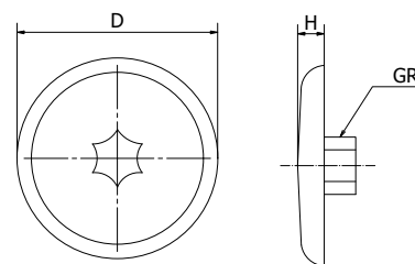
Torx
